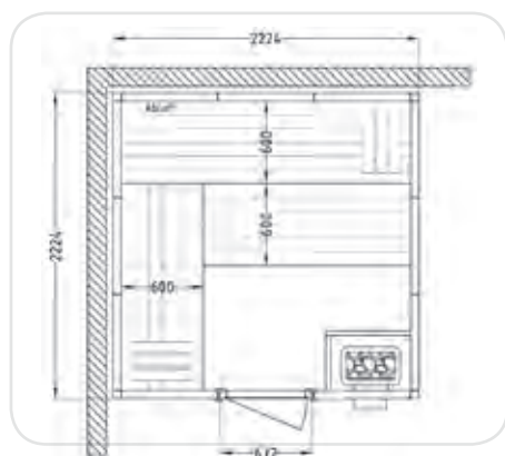
FINESSE Beispiel-Grundriss 222 x 222 cm
