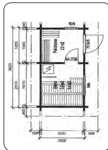
MAALI Sauna Family
