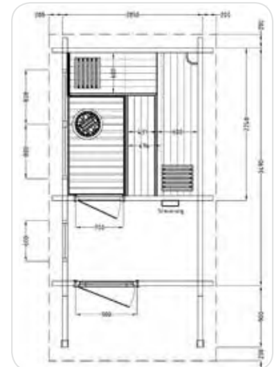
MAALI Sauna Typ 2
