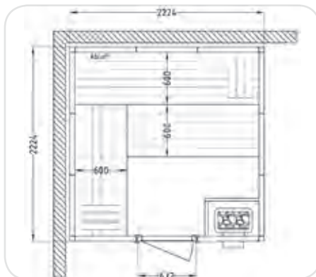
SUPREME Beispiel-Grundriss 222 x 222 cm
