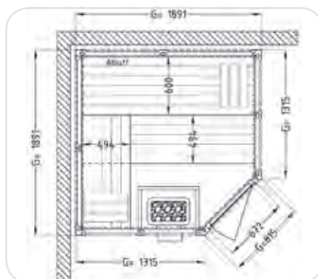
CASA Beispiel-Grundriss 189,1 x 189,1 cm mit EckEinstieg
