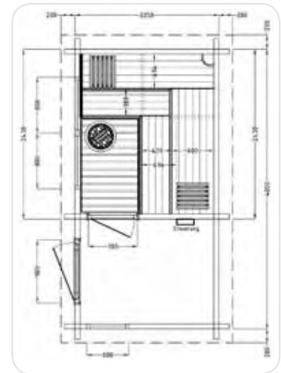
MAALI Sauna Typ 1
