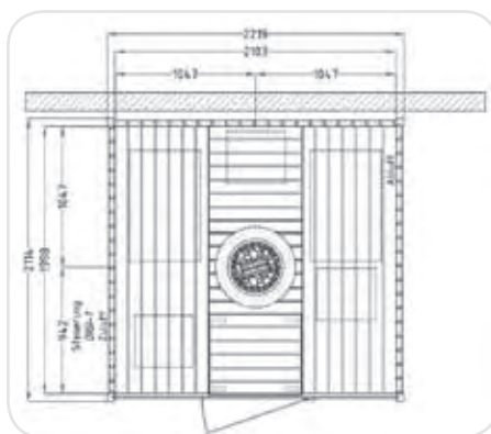
MOCCA Lounge Beispiel-Grundriss 221,9 x 211,4 cm
