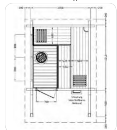
MAALI Sauna Typ 2
