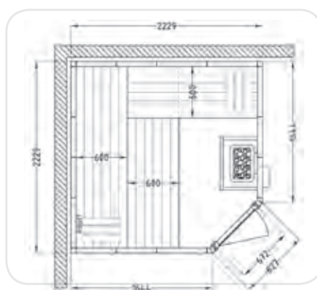
FINESSE Beispiel-Grundriss 222 x 222 cm mit ECKEINSTIEG
