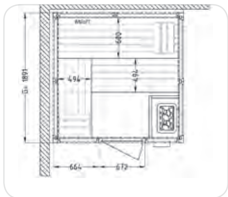
CASA Beispiel-Grundriss 189,1 x 189,1 cm
