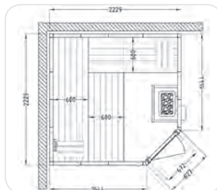
SUPREME Beispiel-Grundriss 222 x 222 cm mit Eckeinstieg
